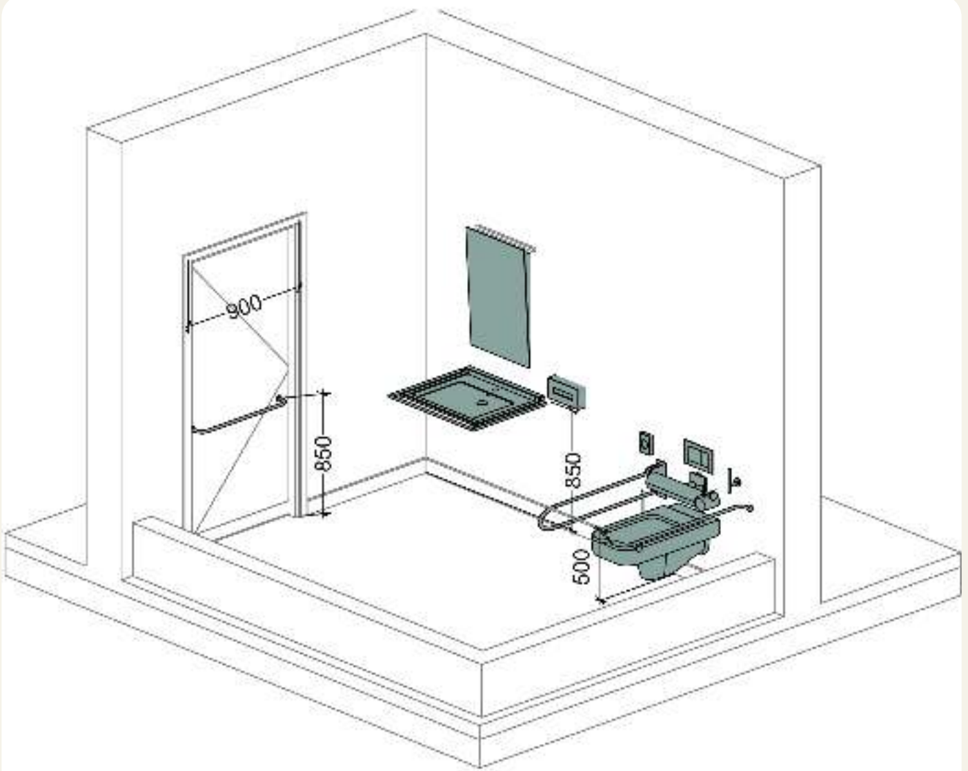
Рис 2. Схематичне зображення окремого санітарно-гігієнічного приміщення для МГН (розміри зазначені у міліметрах)
